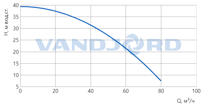
76323707 - VSL.80.75.2.5.0D.T Гидравлическая характеристика
